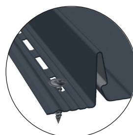
Kruvi õige kinnituspinge tänu mikrosoontele
