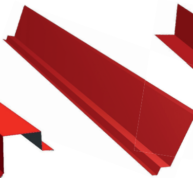
LIITEPLEKK KÜLJELT 40 x 60 x 275 mm, L=2 000 mm
