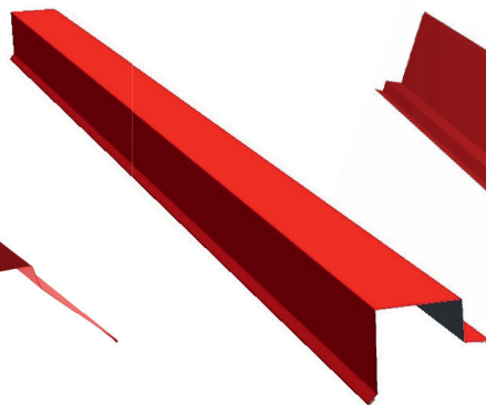
VIILUPLEKK 87 x 80 x 40 mm, L=2 000 mm
