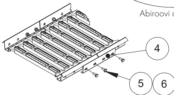
Kinnitus 50 x 100 mm abiroovi külge 7 x 50 mm kruvidega.
